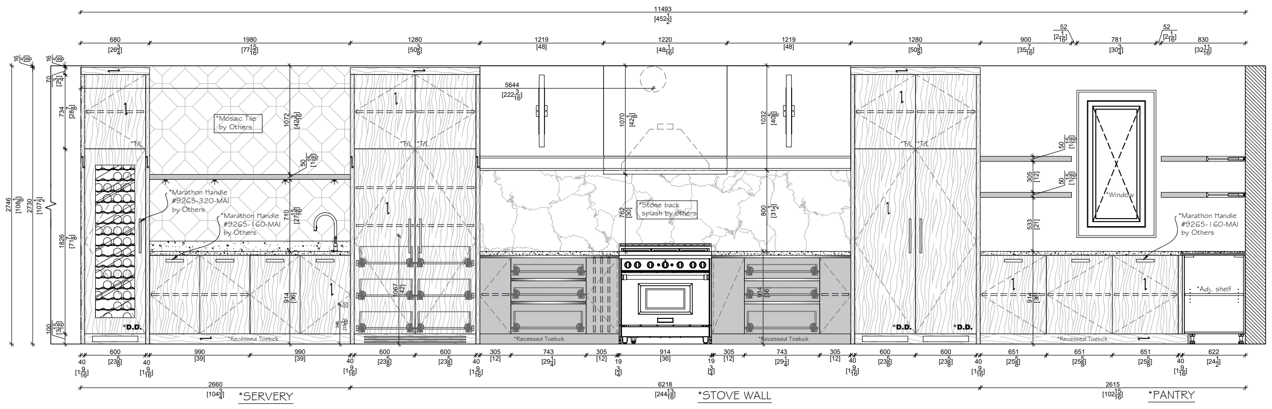
ELEVATION A SCALE: 1:25
