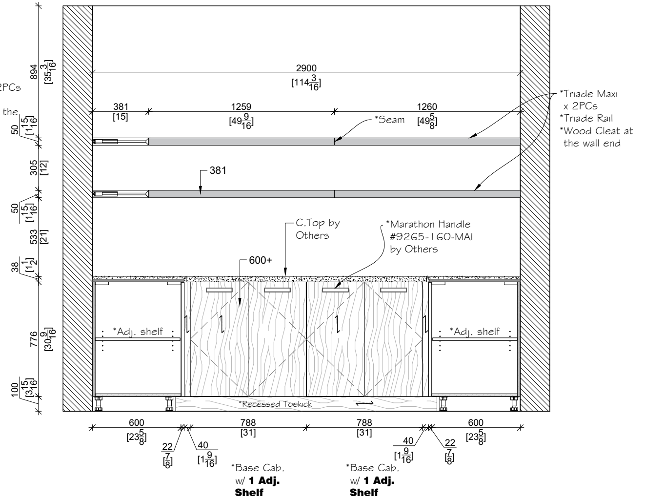
ELEVATION C SCALE: 1:25
