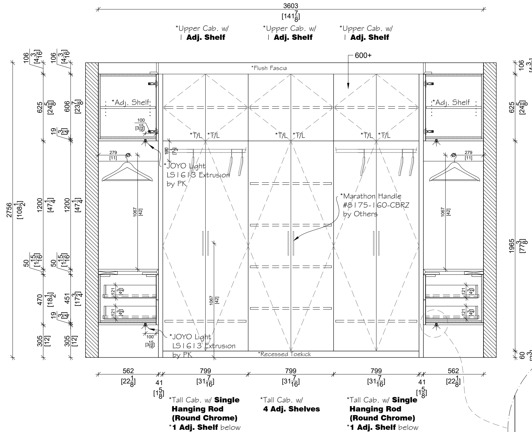
ELEVATION B SCALE: 1:22
