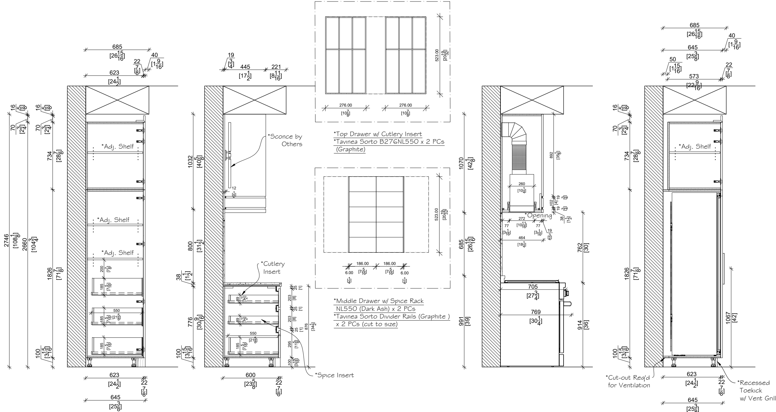
S5-SECTION SCALE: 1:25
