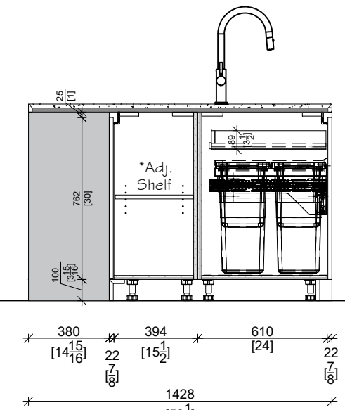
S8-SECTION SCALE: 1:25
