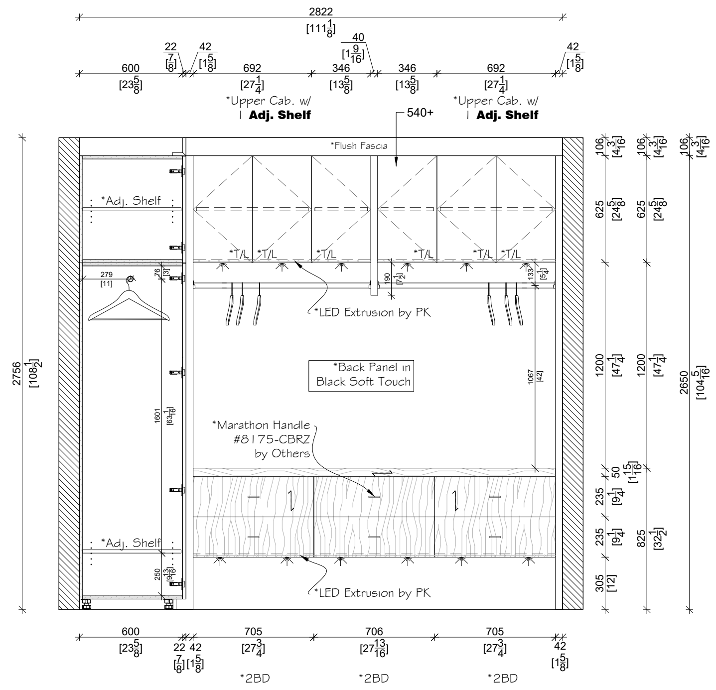
ELEVATION C SCALE: 1:22
