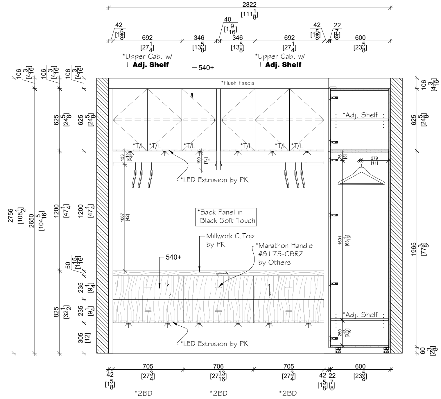
ELEVATION A SCALE: 1:22
