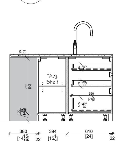
S8-SECTION SCALE: 1:25
